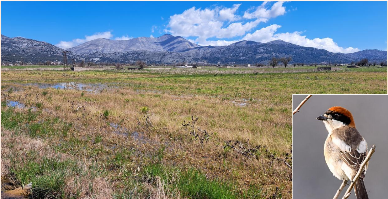
Lasithi-Hochebene, Rotkopfwürger
